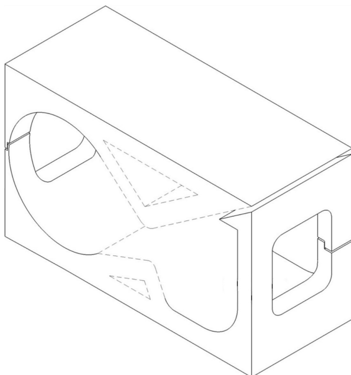
2. Зажим медицинский для трубок с замками-защёлками (вариант 2)
